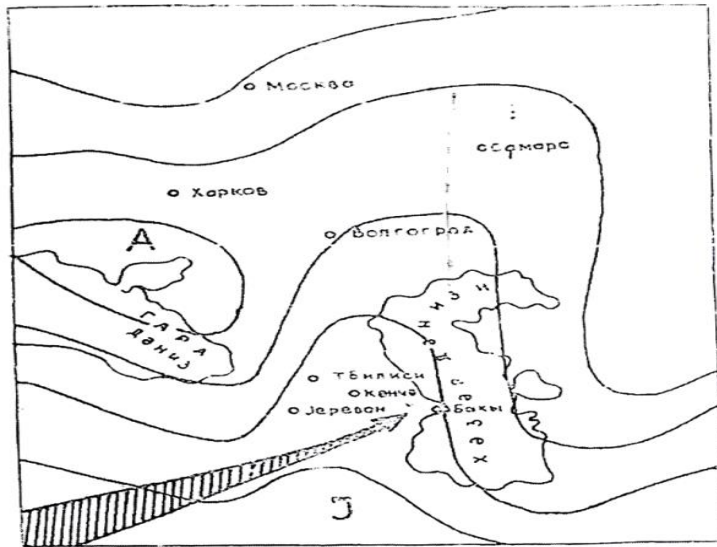
Şəkil 3. Tropik hava kütlələrinin daxil olması
