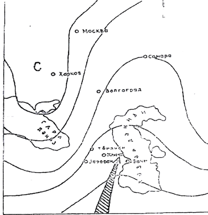
Şəkil 4. Cənub siklonlarının daxil olduğu ərazi
