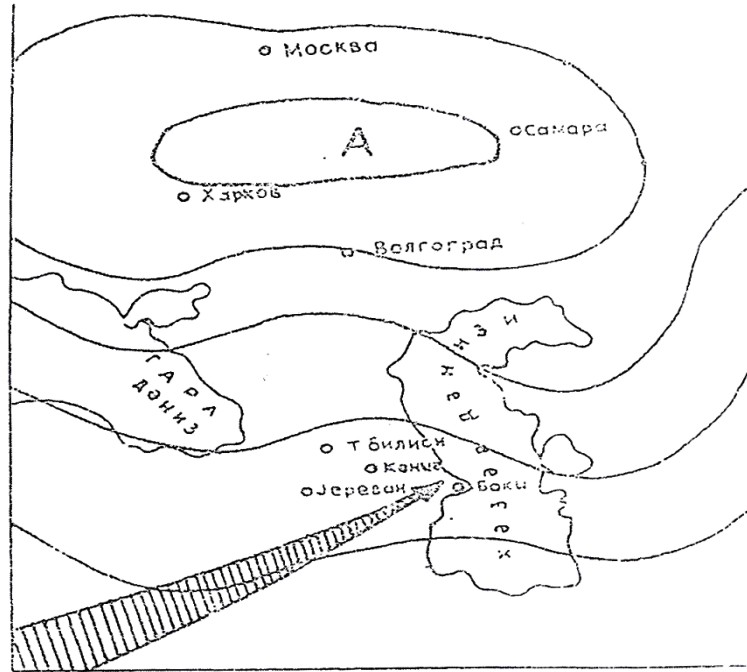
Şəkil 1. Yerli atmosfer prosesləri
