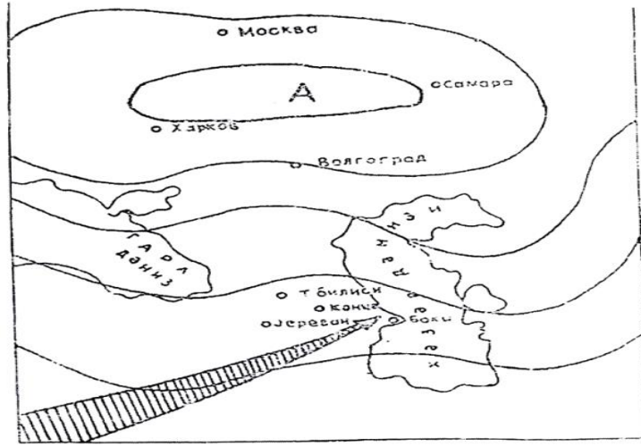
Şəkil 2. Tropik hava kütlələrinin daxil olması
